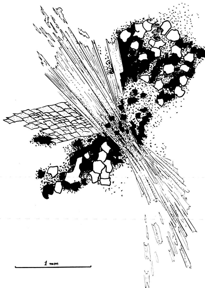
FIG 60 (pl. m. 93 V). — Faisceau de longs prismes d'amphibole de couleur bleu-violacé pâle, se développant dans un fond gréseux et microbréchique. Localement, forte pigmentation rousse et opaque.
