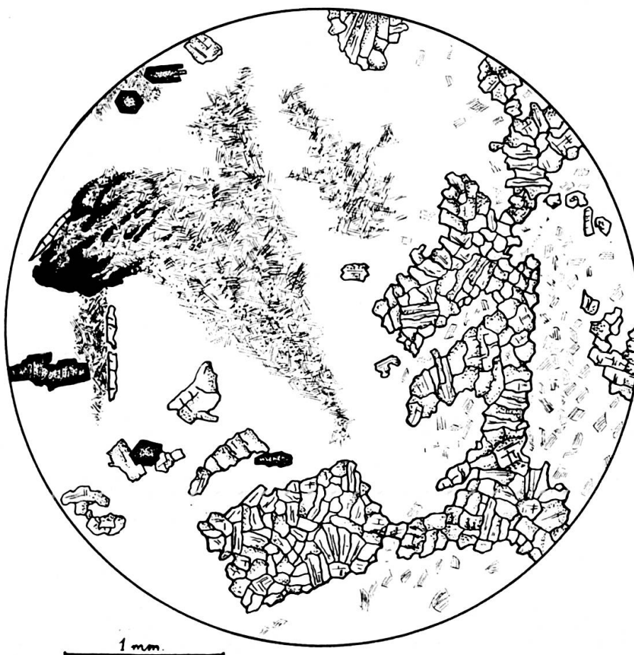
FIG. 41 (pl. m. 72 V). — Gabbro à phénocristaux de plagioclase nombreux. La zone interstitielle triangulaire, entièrement chloritisée et amphibolisée, avec mica et stilpnomélane ou biotite (vert). Les phénocristaux de plagioclase sont transformés en albite, variété d'épidote, phyllite; présence de tourmaline et de deux petites aiguilles d'apatite. Grain d'ilménite déformé et altéré.
