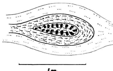
FIG. 1 (plaque mince 1 V). Lumière naturelle. — Structure microscopique idéalisée de variolo de « coussin » très faiblement métamorphique, légèrement laminée (Prainan).
