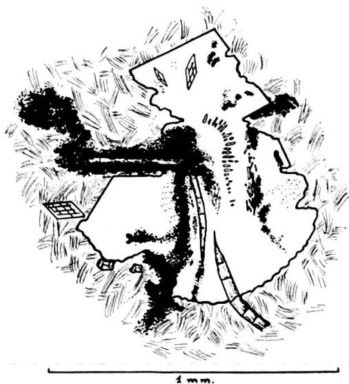
FIG. 4 (pl. m. 2 V). — Idem que fig. 2 et 3. Un prisme amphibolique, parallèle à une trainée semi-opaque, est brisé et inclus dans un phénoblaste d'albite.
