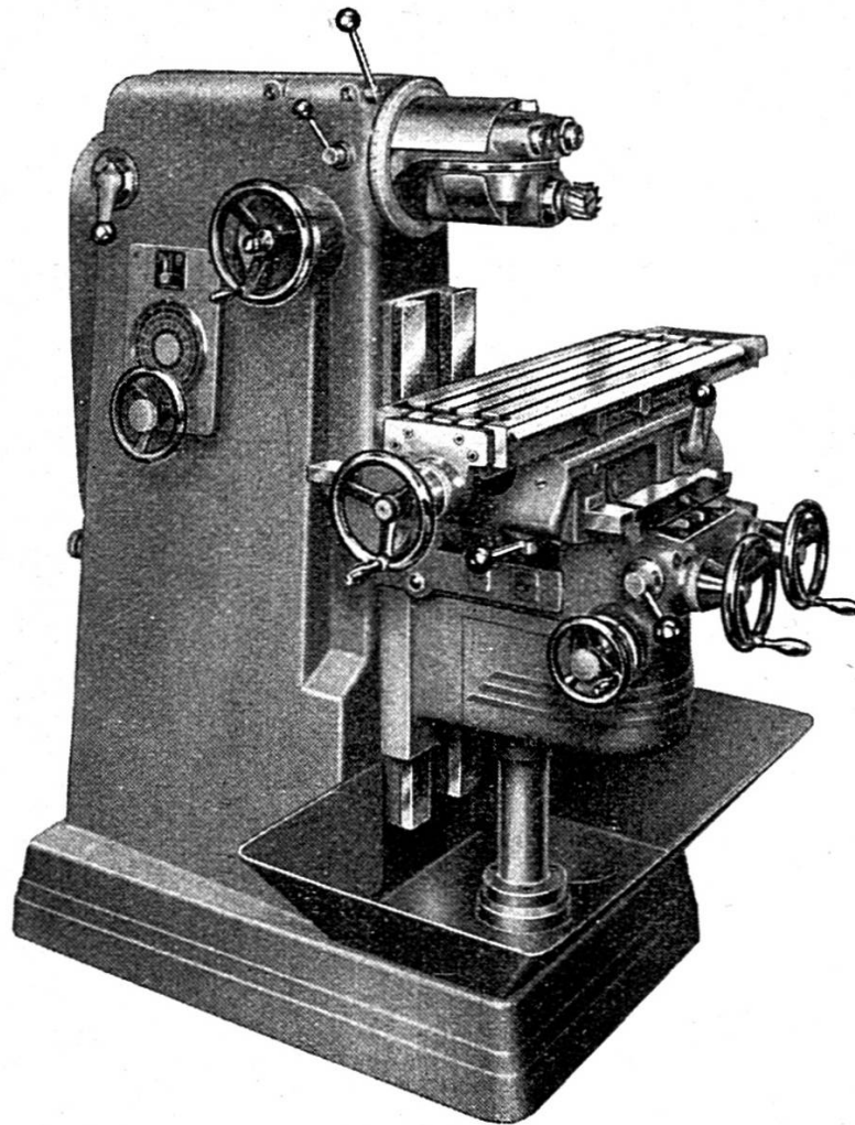
Fraiseuses universelles de grande précision SV 51 / SV 53 Surface de la table 800×215 1100×255 mm
