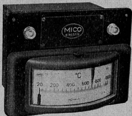
Régulateur électronique de température pour thermo-couple Hoskins Etendue de mesure : 20 — 1000° C
