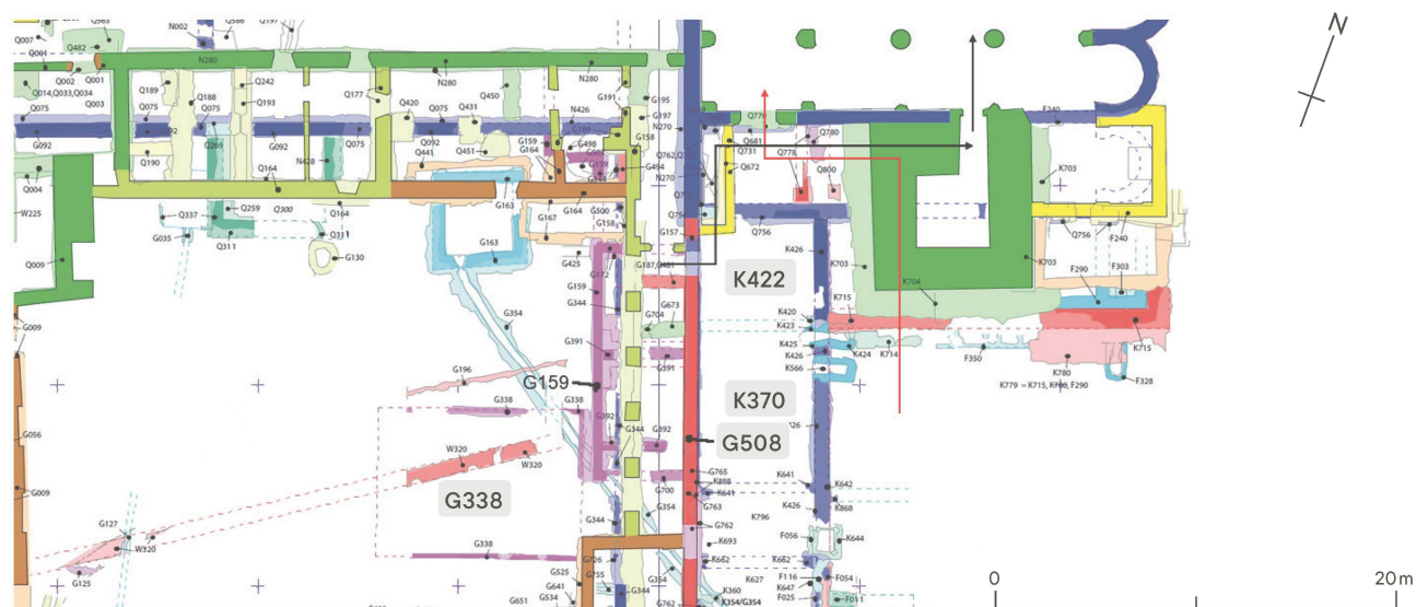
Abb. 5: Münstair, Plan der archäologischen Befunde mit Positionsnummern und Bauphasen: Ausschnitt Ostflügel mit Zugangswegen zur Kirche. Mst. 1:400.
