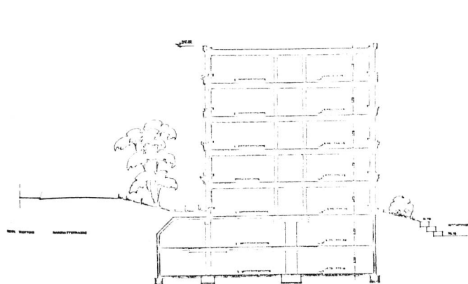
SCHNITT A-A
