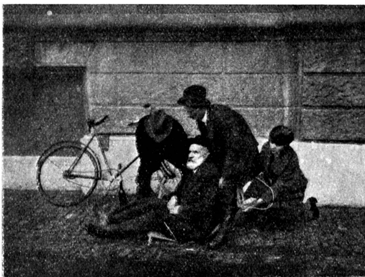
Fig. 3. Deuxième temps: glissez le sac sous le siège du blessé.
