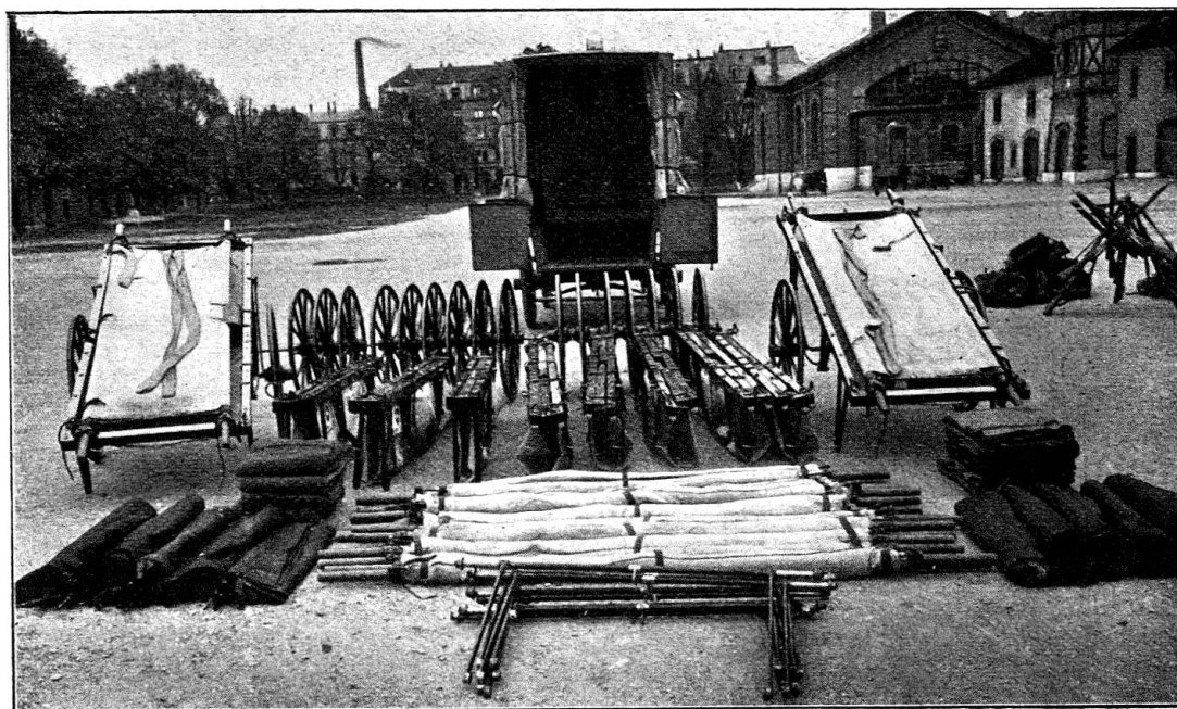
Fig. 3. Contenu du fourgon; deux branchards-roulants sont montés à droite et à gauche de la planche.
