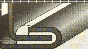
Falzverdichtung und Feinabdichtung.
