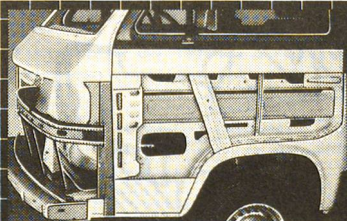
Eingebaute Sicherheits-Verstrebungen
