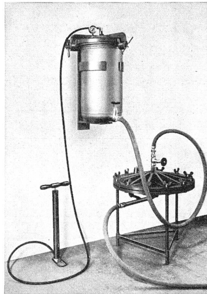
Einschichtenfilter mit Druckgefäß für Kleinfiltrationen
