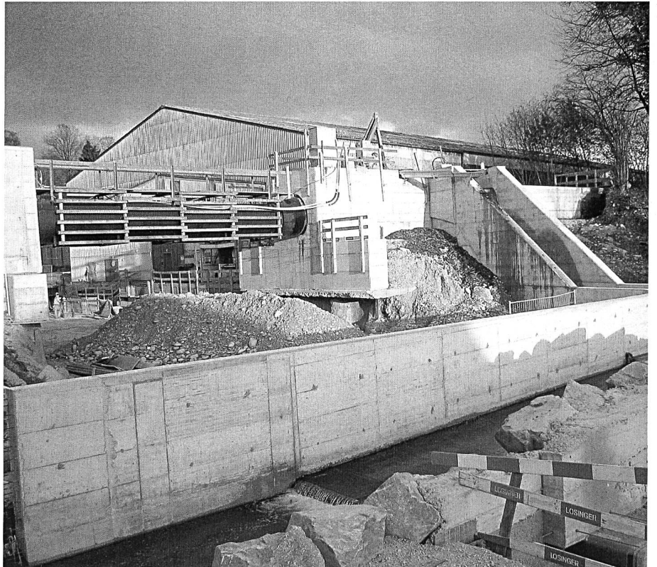
Die Überleitung des Tych und das Wasserschloss des Kleinkraftwerks Wäbi.
