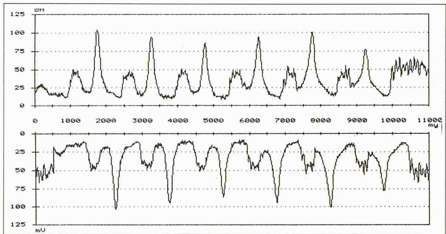
Bild 10. Analoges Abstandssignal der beiden faseroptischen Taster eines Innengewindesensors über sechs Gewindengänge (Quelle: FhG-IPT, Aachen)
