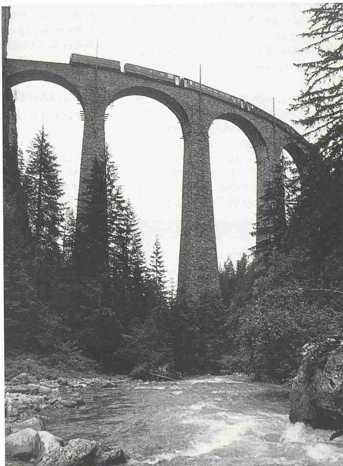
Der Landwasserviadukt bei Filisur auf der Albulalinie (eröffnet 1903). Der kühne Viadukt hat einen Radius von 100 m, ist 130 m lang, 65 m hoch, hat sechs Bogen mit 20 m Spannweite und mündet direkt in eine senkrechte Felswand ein
