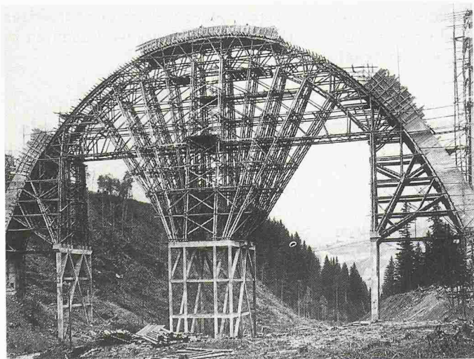
Das Lehrgerüst des Langwieser Viadukts zwischen Chur und Arosa (um 1912). Die erste derartige Eisenbetonkonstruktion der Schweiz, 287 m lang, 62 m hoch, der Mittelbogen mit 96 m Spannweite (Bilder: RhB)
