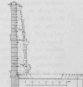
Abb. 4. Schnitt A-B. 1 : 300.
