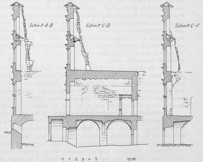
Abb. 3. Schnitte. — Masstab 1 : 300.
