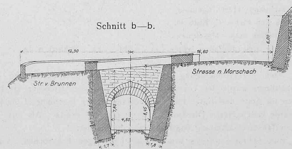
Abb. 10. Gewölbte Strassen-Ueberführung bei Km. 0,71. Masstab 1 : 400.
