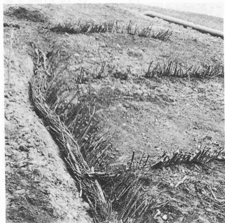
Bild 13. Kerzers N1. Aus dem Hang austretendes Wasser wurde mittels Bündelfaschinen in Ypsilon-Dränen abgeleitet (biotechnische Entwässerung)
