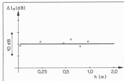
Diagramm 3. Abhängigkeit der Schalldämmung von der lichten Abhängehöhe h bei leerem Hohlraum.
