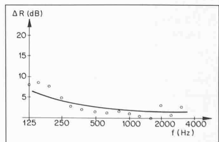
Diagramm 7. Differenz in der Schalldämmung zwischen einem offenen und einem geschlossenen Hohlraum mit 50 mm Mineralwolle-Auflage. Abhängehöhe: 610 mm.
