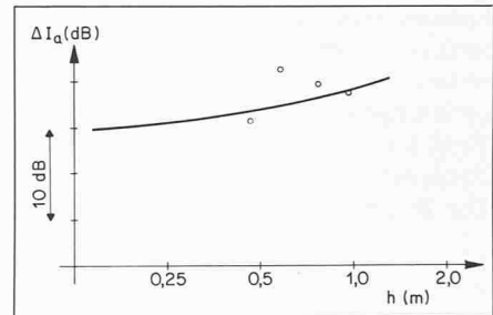
Diagramm 5. Abhängigkeit der Schalldämmung von der lichten Abhängehöhe h bei leerem Hohlraum.
