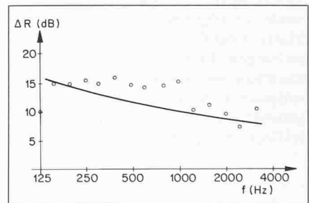
Diagramm 6. Differenz in der Schalldämmung zwischen einem offenen und einem geschlossenen Hohlraum. Deckenhohlraum ungedämpft bzw. leer. Abhängehöhe: 610 mm.
