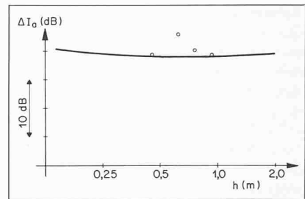
Diagramm 4. Abhängigkeit der Schalldämmung von der lichten Abhängehöhe h bei 50 mm Mineralwolle-Auflage.
