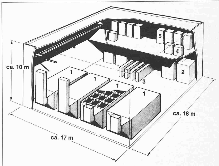
Bild 6. 13,6 MWh-Na/S-Batteriespeicherwerk
