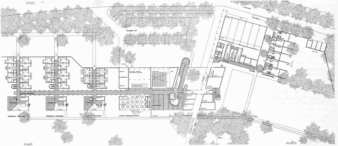
Grundriss Erdgeschoss 1:1200
