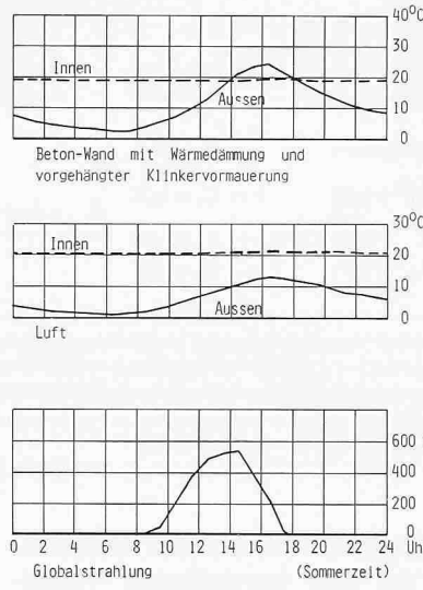
Bild 5. Messungen Südwestseite: Temperaturen und Einstrahlung am 24. April 1981
