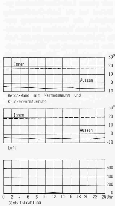
Bild 8. Messungen Südwestseite: Temperaturen und Einstrahlung am 17. Jan. 1980
