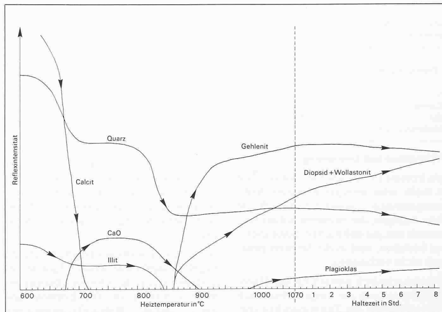
Bild 6. Verlauf der Reflex-Intensitäten aus der Röntgendiffraktometeraufnahmen mit Heizkamera. Aufheizen des Dachziegelrohmaterials 1^\circ\text{C}/\text{min}
