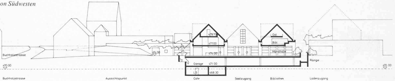
Schnitt Café/Bibliothek
