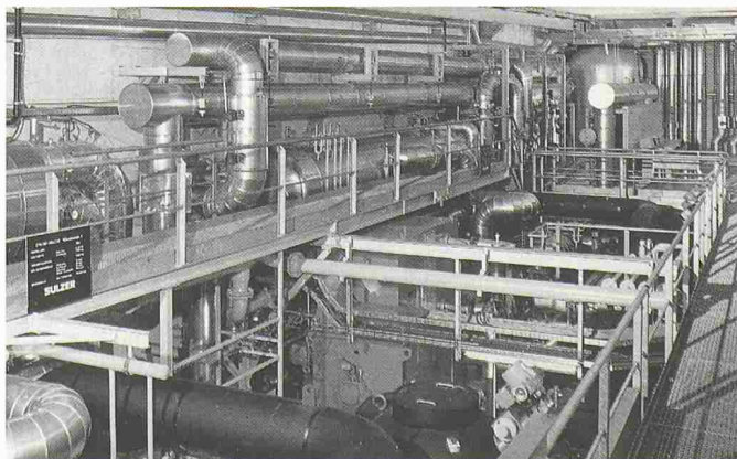
ETH-Wärmepumpenanlage Walche
