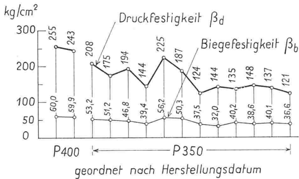
Bild 23. Mörtelfestigkeiten an 4×4×16 cm Prismen eingesandt von Baustelle Wohnhochhäuser «Altwyler» in Bern. Sinkende Mörtelfestigkeiten mit abnehmender Beanspruchung des Mauerwerkes
