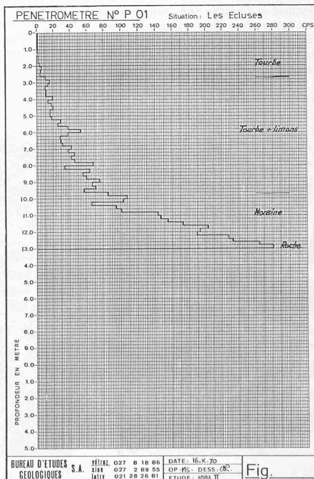
Fig. 8. — Résultats des sondages au pénétromètre.
