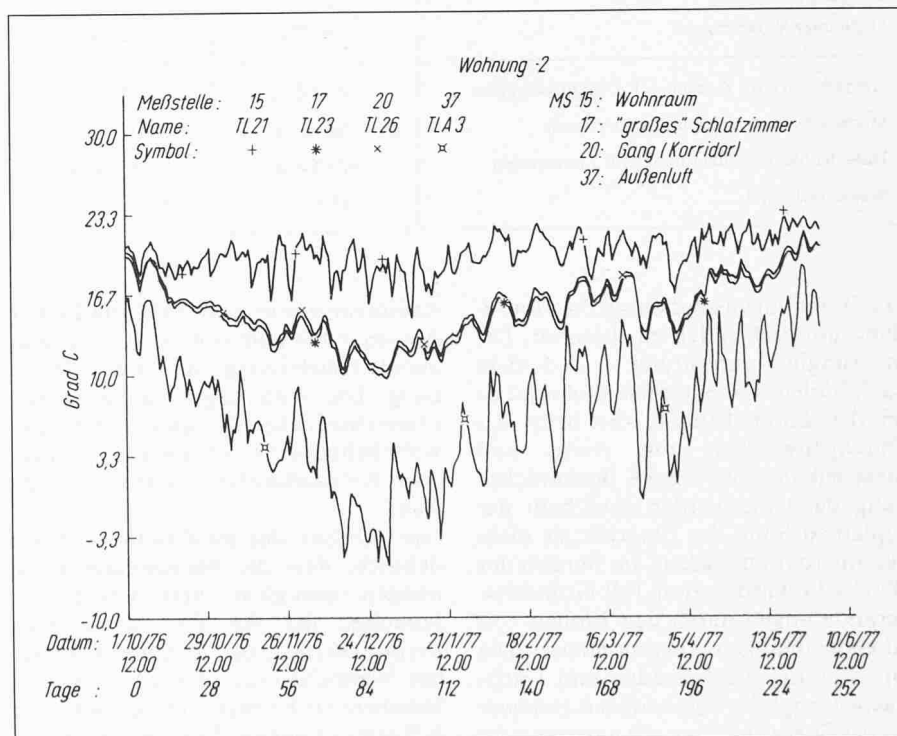
Bild 2. Auswertung der Tagesmittelwerte der Wohnung 2 in der Messperiode November 1976 bis Juni 1977. Die Abweichung der mittleren Wohnungstemperatur von 18^\circ\text{C} beträgt \pm 1,5\text{ K} je nach Bewohner; dadurch entstehen Extreme des Heizenergieverbrauches im gleichen Haus von bis zu 1:6. Die Wohnraumtemperaturen liegen bei 20,5^\circ\text{C} \pm 0,5\text{ K} , die Schlafräume werden dagegen weniger beheizt, so dass eine Absenkung der mittleren Wohnungstemperatur während der Winterspitze entsteht. Dadurch reduziert sich die benötigte Heizleistung der Zimmeröfen um rund 20%
