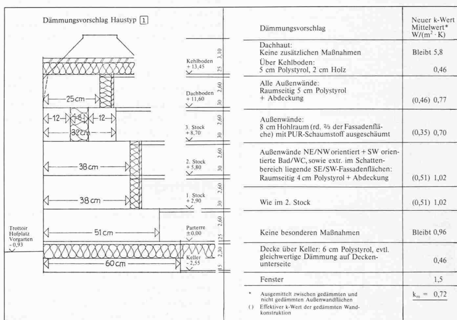
Bild 4. Schema der Wärmedämmung Typ 1. k -Wert verbessert auf 0,72 \text{ W}/(\text{m}^2 \cdot \text{K}) für k_m . Die spezifische Heizleistung beträgt nur noch 71 \text{ W}/\text{K} je Wohnung
