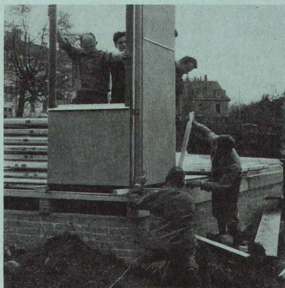
Das Trelement-Haus in der Montage. Architekt: Eberhard G. Rensch, Frankfurt am Main
