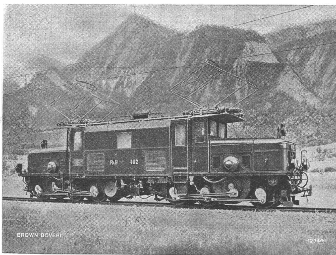
Einphasenstrom-Lokomotive, Typ C-C für die Rhätische Bahn 2 × 600 PS, 10 000 Volt Fahrdrachtspannung, Frequenz 16 2/3 Geschwindigkeit 30 bis 45 km/h, Spurweite 1 m.
