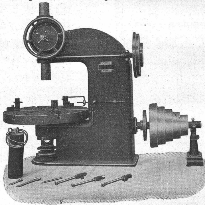
Riemenscheiben-Ausbohrmaschine.
