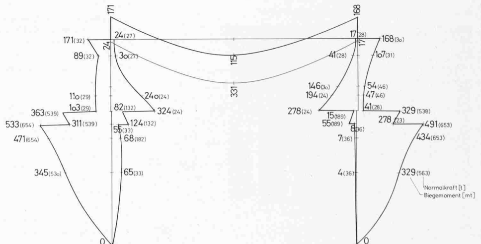
Bild 8. Grenzwertlinien Haupttrahmen
