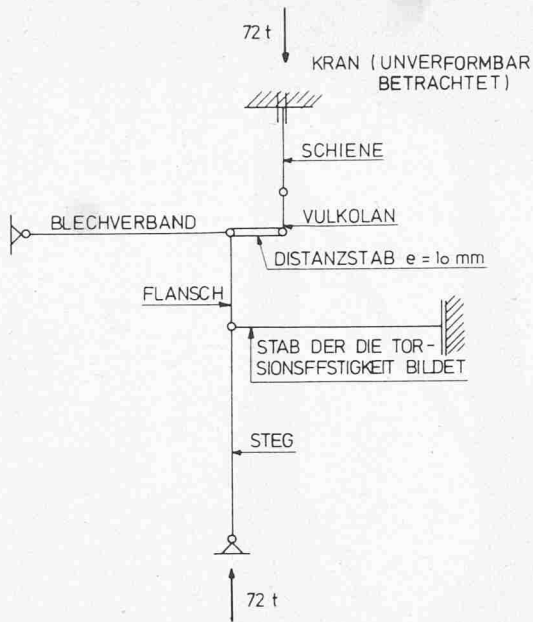
Bild 12 (oben). Stabmodell
