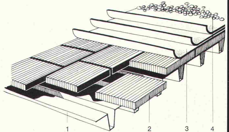
METALLPROFILDACH
