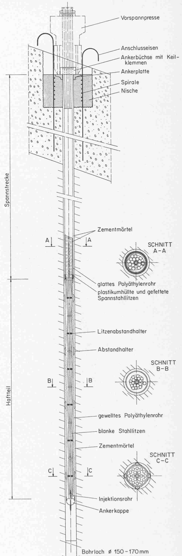
Bild 6. VSL Felsanker
