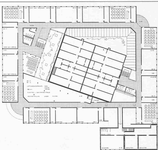
1. Untergeschoss
