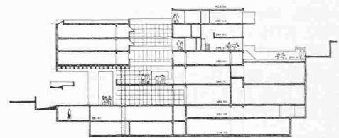
Schnitt 1-1, 1:1000
