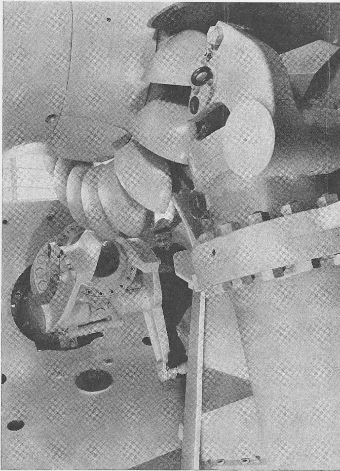
Bild 8. Blick ins Innere des Turbinengehäuses mit den beiden Einläufen
