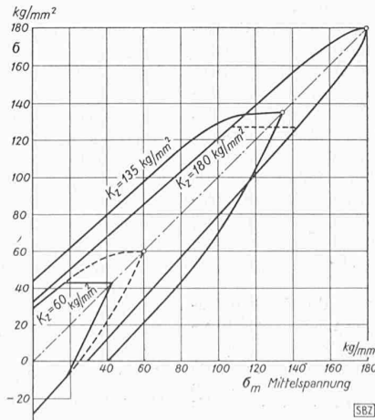
Abb. 3. Wöhlerlinie Abb. 2 (links). Dauerfestigkeit für Biegung von Seildrähten, nach Versuchen im Kaiser Wilhelm Institut für Eisenforschung in Düsseldorf (nach «Glückauf» 1941, S. 261/62)
