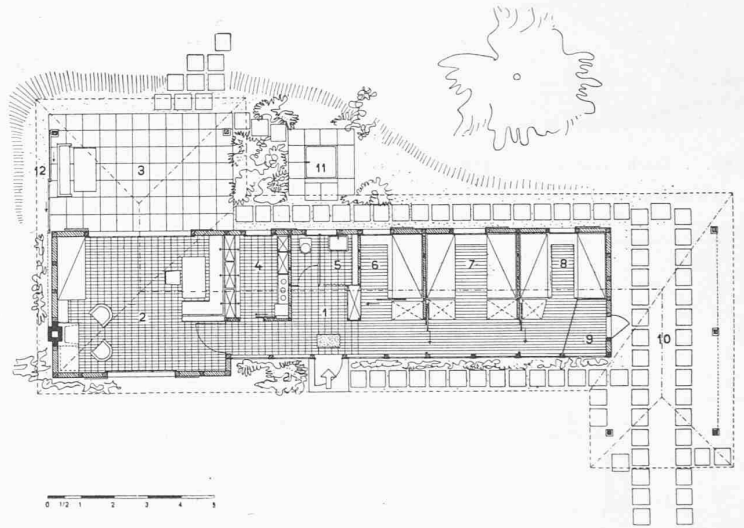
Abb. 1. Grundriss, Masstab 1 : 200. — Legende im Text
