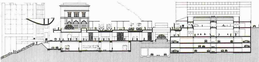
Sezione trasversale
