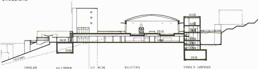
Sezione trasversale
