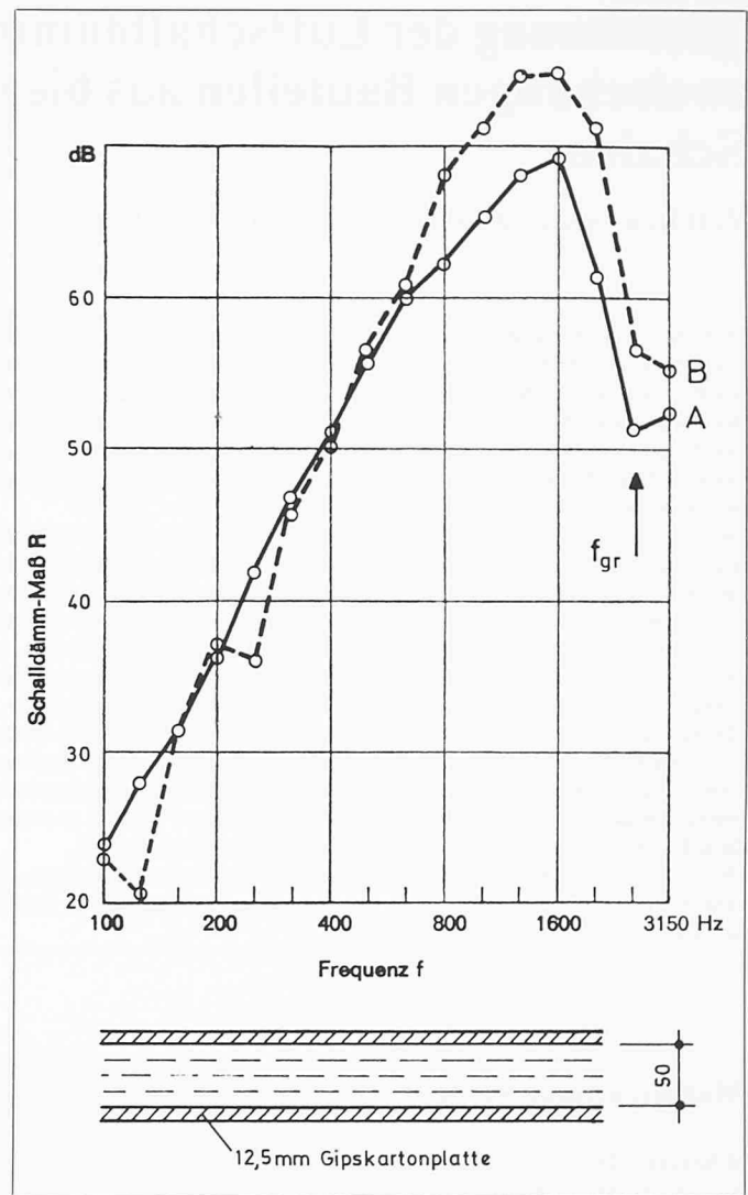
Bild 2. Luftschalldämmverlauf einer zweischaligen Trennwand aus Gipskartonplatten (Aufbau wie im vorigen Beispiel) Kurve A: Messkurve. Kurve B: berechnet nach Formel (4)
