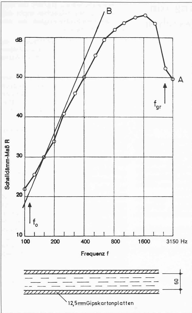
Bild 1. Luftschalldämmverlauf einer zweischaligen Trennwand aus Gipskartonplatten Kurve A: Messkurve. Kurve B: berechnet nach Modell
