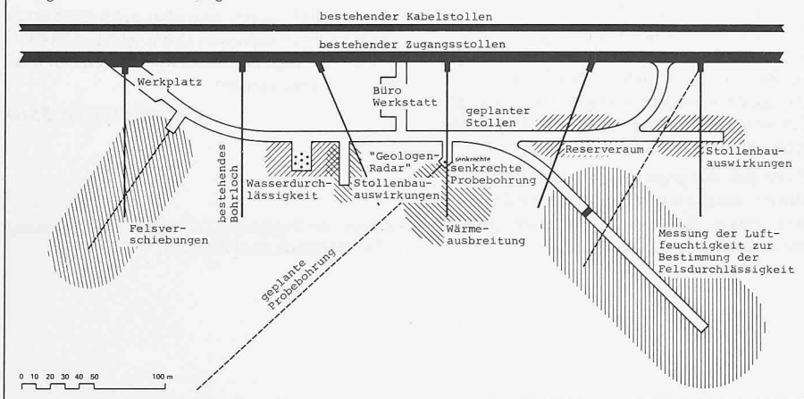
Nagra-Versuchslabor: möglicher Grundriss
