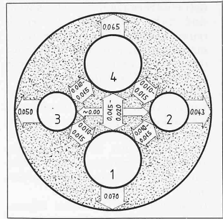
Bild 10. Wärmeverlustfaktoren in [W/m K]
