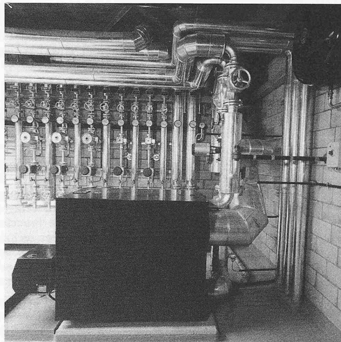
Bild 7. Spitzheizkessel. Heizleistung 110 kW
