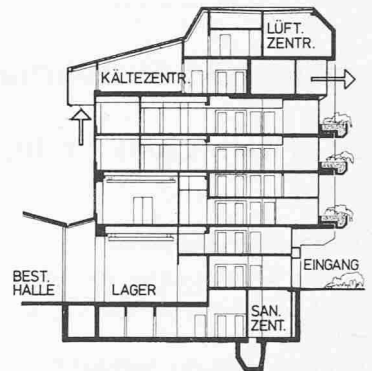
Schnitt Eingangspartie 1:750
