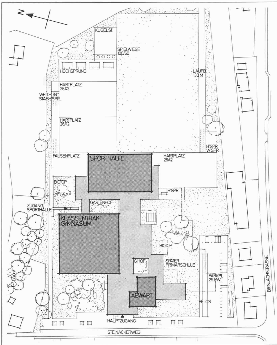
Lageplan 1:1750
