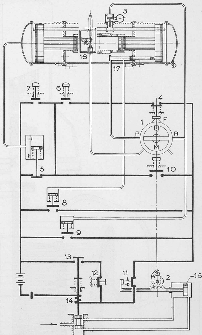
Bild 5. Steuerschema eines Gaserzeugers. 1 Handrad des Steuerapparates, 2 Hydraulische Vorrichtung zur Betätigung des Steuerapparates, 3 Anlasseluftzwischenbehälter, 4-13 Steuerkontakte, 14 Magnetspule, 15 Steuerkolben, 16 Pneumatische Stopvorrichtung, 17 Pneumatischer Kolbenversteller
