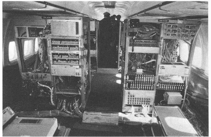
Équipement aéroporté de télémessure en temps réel.
