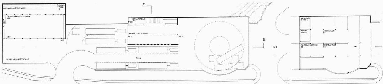
Grundriss Feuerwehrstützpunkt und Busgarage 1:900
