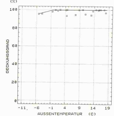
Anteil Wärmelieferung der WP am Gesamtwärmebedarf, Messdaten 1984-1986
