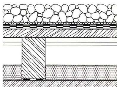
Kaldach Beispiel: Isolierung auf Stahlbetondecke
