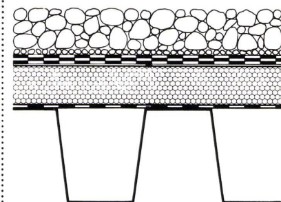
Warmdach Beispiel: Isolierung auf Trapezblechen
