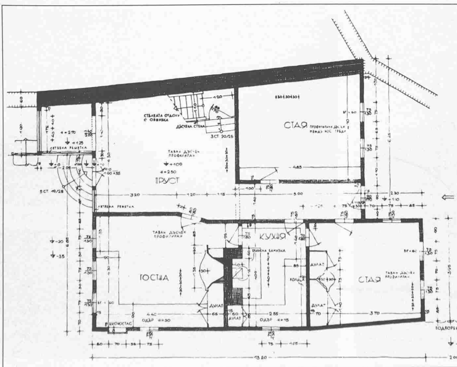
Haus Markov. Grundriss
