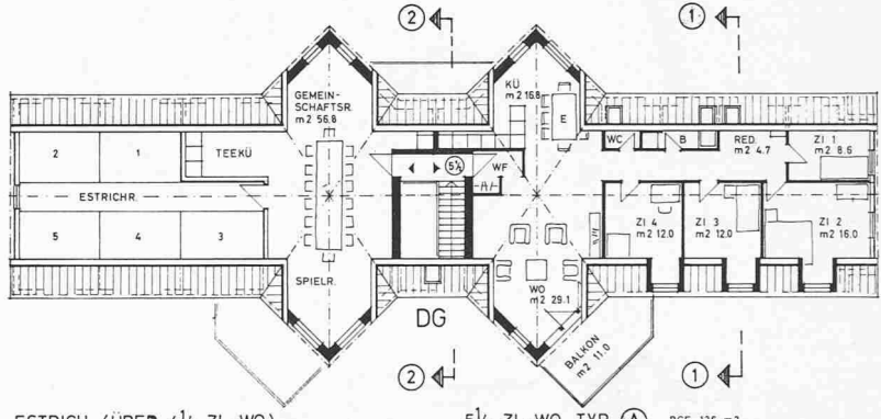
Grundriss-Typen 1:330
